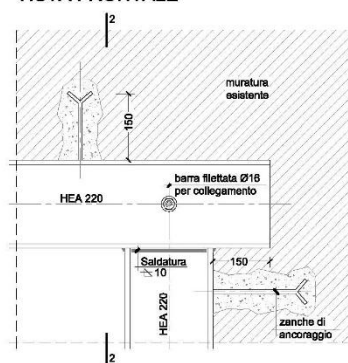
PARTICOLARE "B" 1:10
