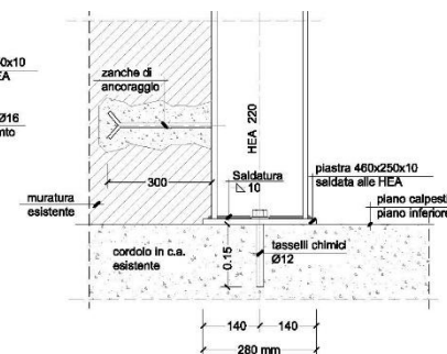
SEZIONE 2-2
